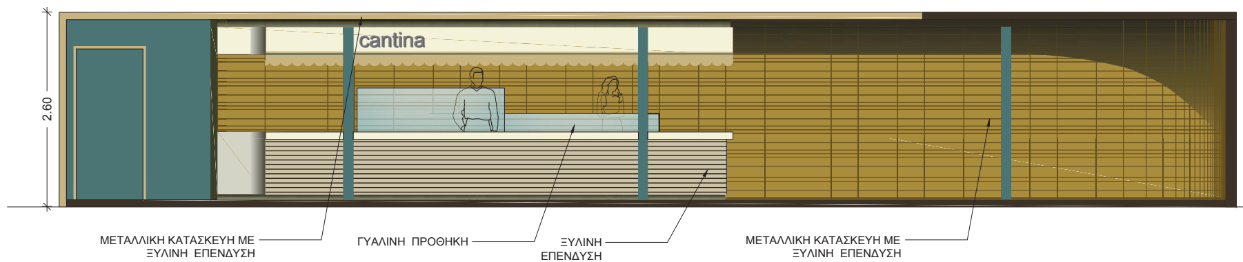
ΟΨΗ ΚΛ.1:50
