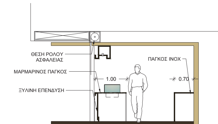
ΤΟΜΗ Α-Α ΚΛ.1:50
